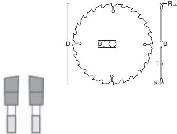
geometrie zubu – střídavé zuby
